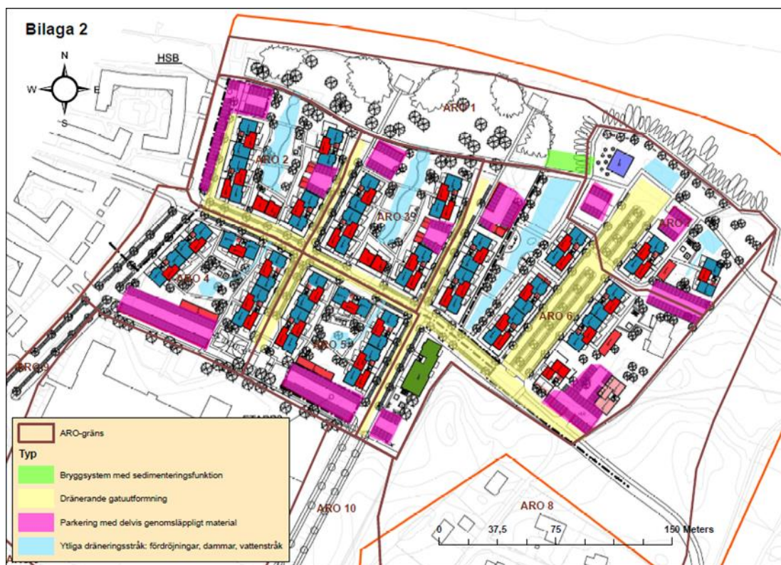
Principskiss, dagvattenstrategi.
